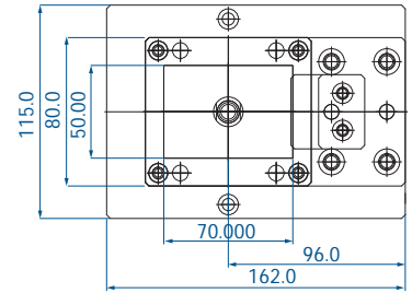
□ 75.0×50.0 金型
